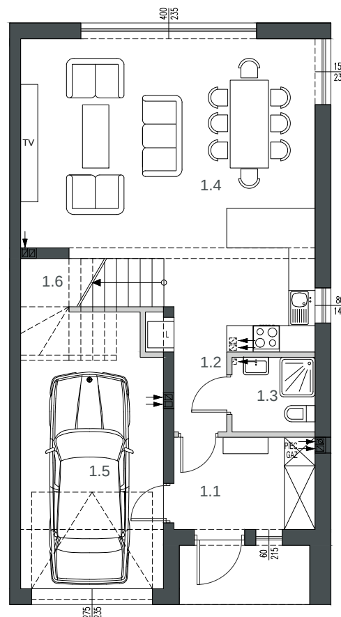
RZUT PARTERU
