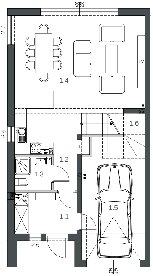
RZUT PARTERU
