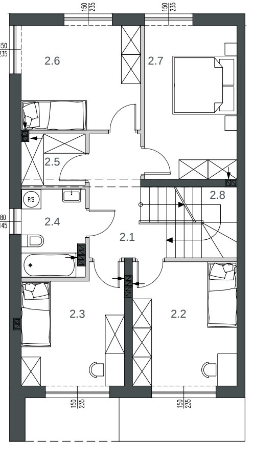
RZUT PIĘTRA
